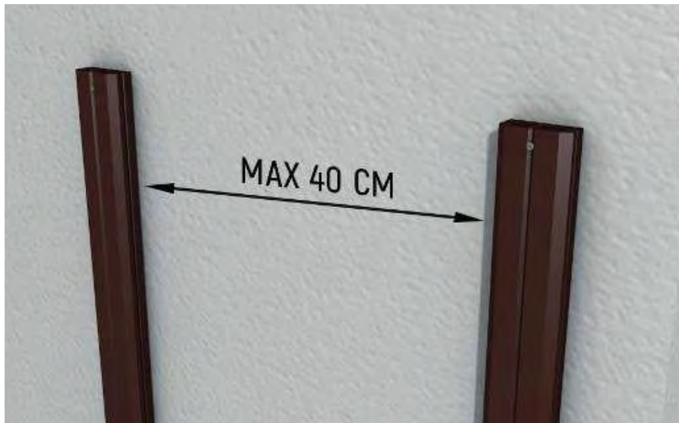
АЛЮМИНИЕВЫЙ ПРОФИЛЬ
